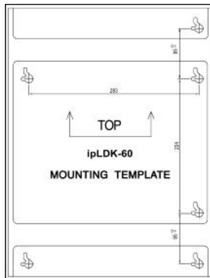
Трафарет для настенного крепления
