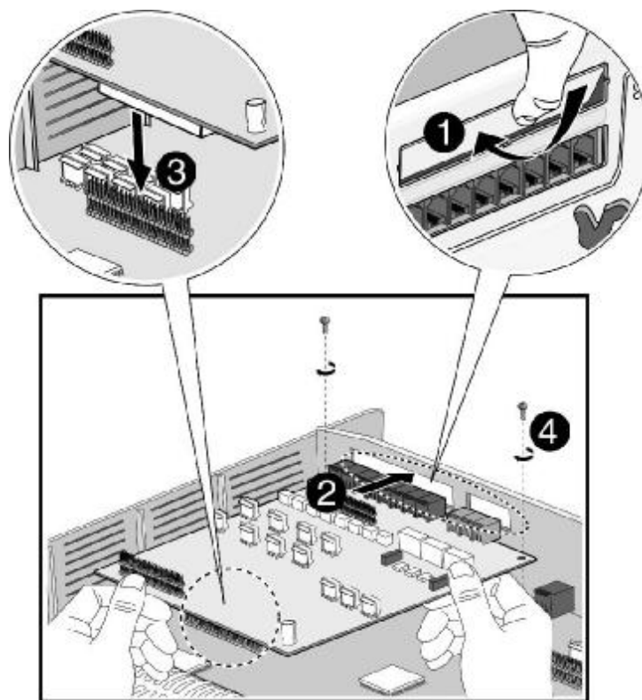
Рис. 4.1 Установка платы
