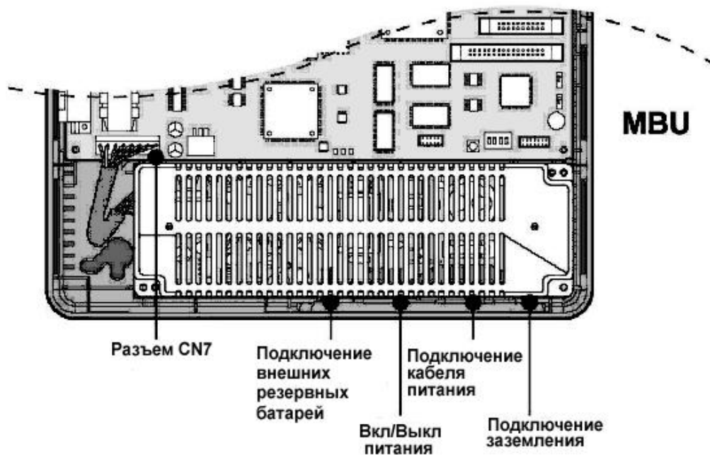
Рис. 3.2.4 Установка блока питания
