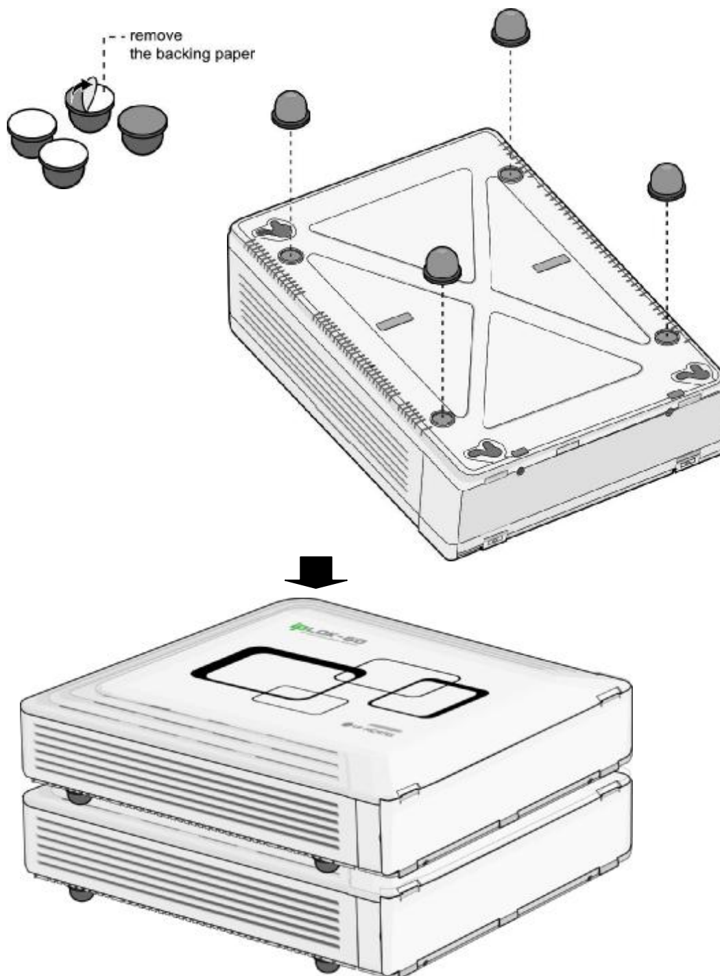
Рис. 3.2.7.3 Настольная / напольная установка
