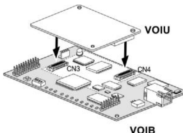
Рис. 4.4.5 VOIU
