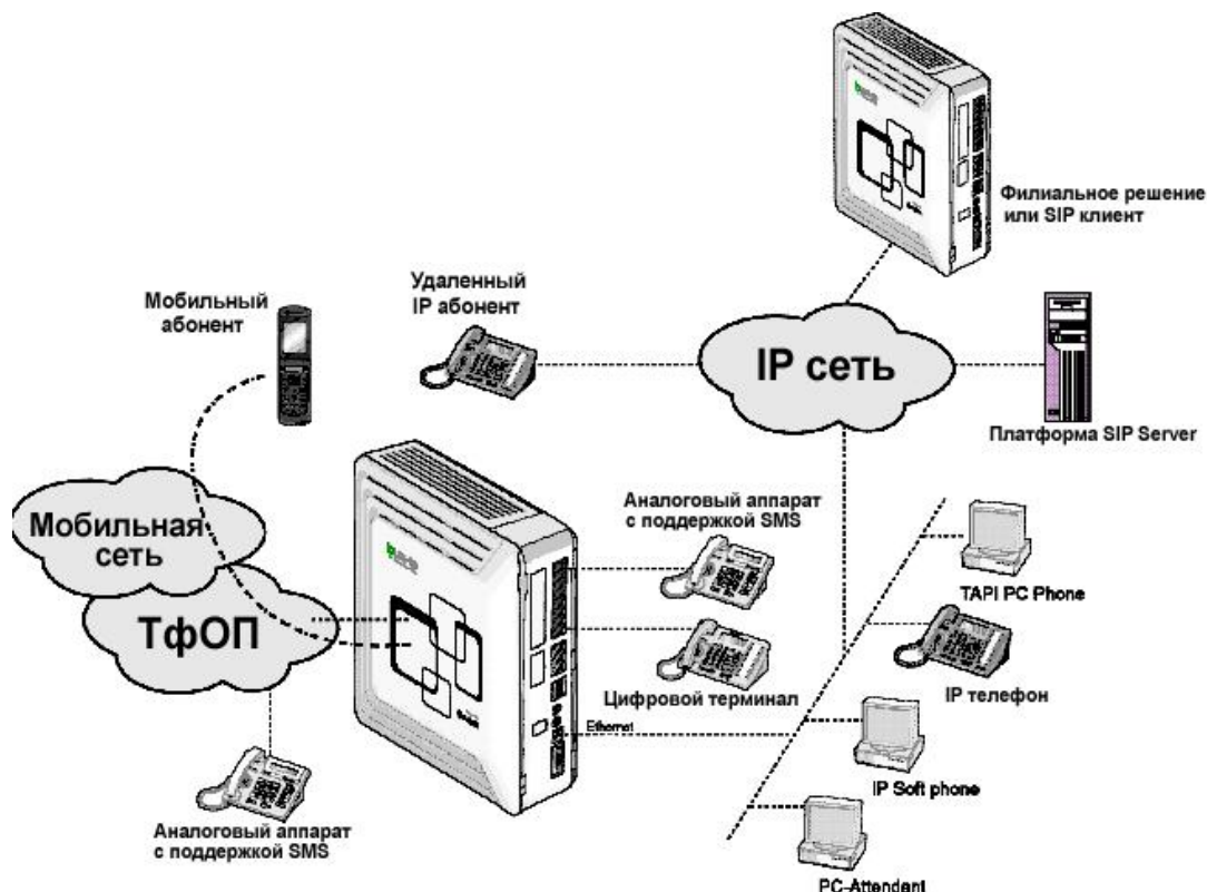
Рис. 2.1.1 Схема подключений
