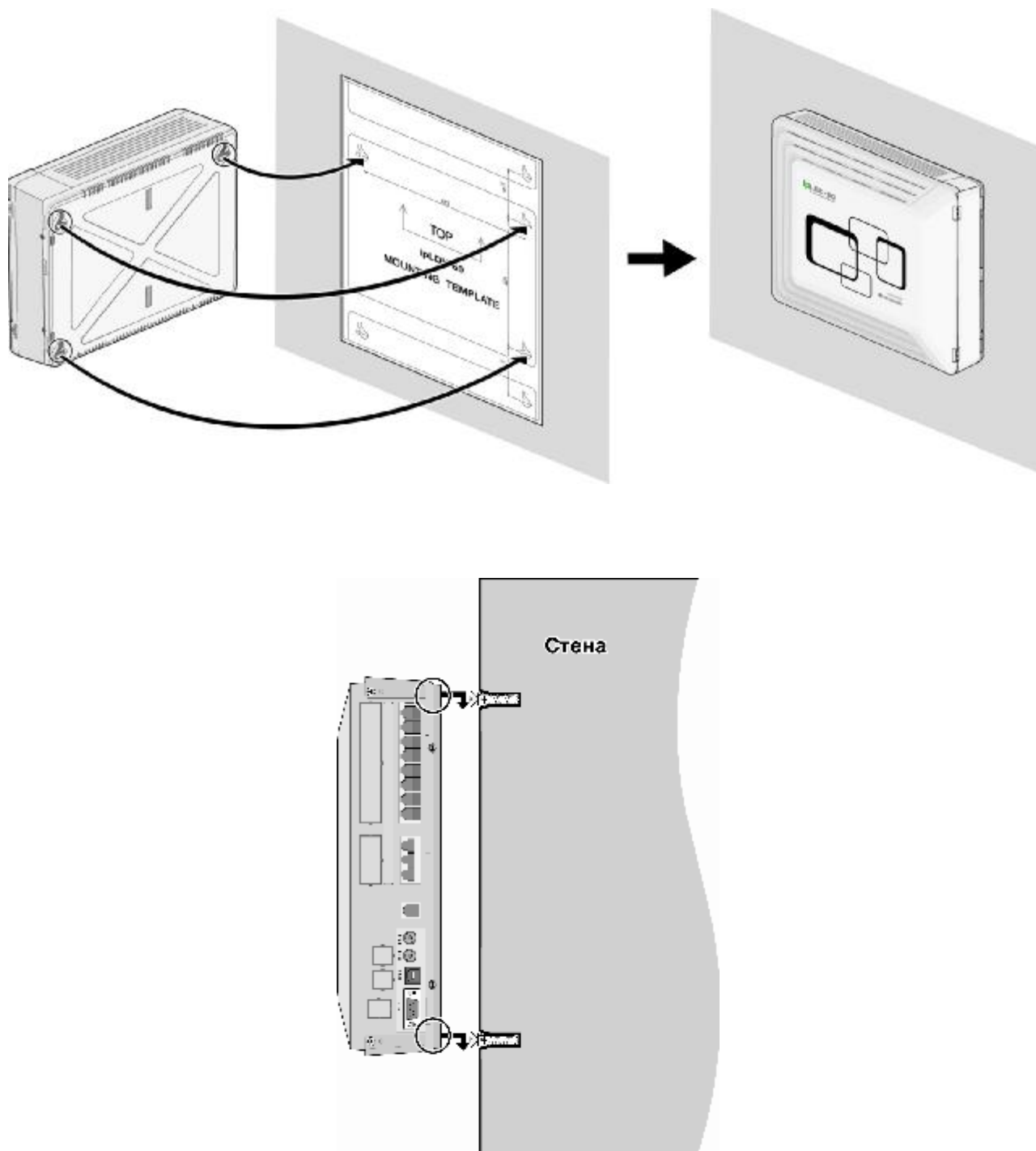
Рис. 3.2.7.16 Настенный монтаж системного блока
