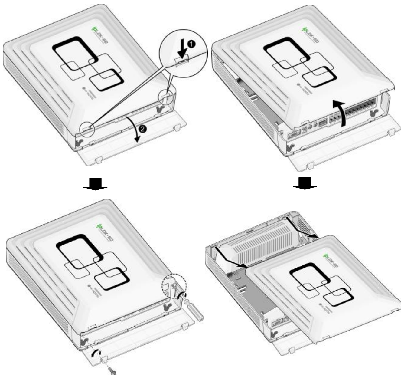
Рис. 3.2.3.1 Снятие лицевой панели
