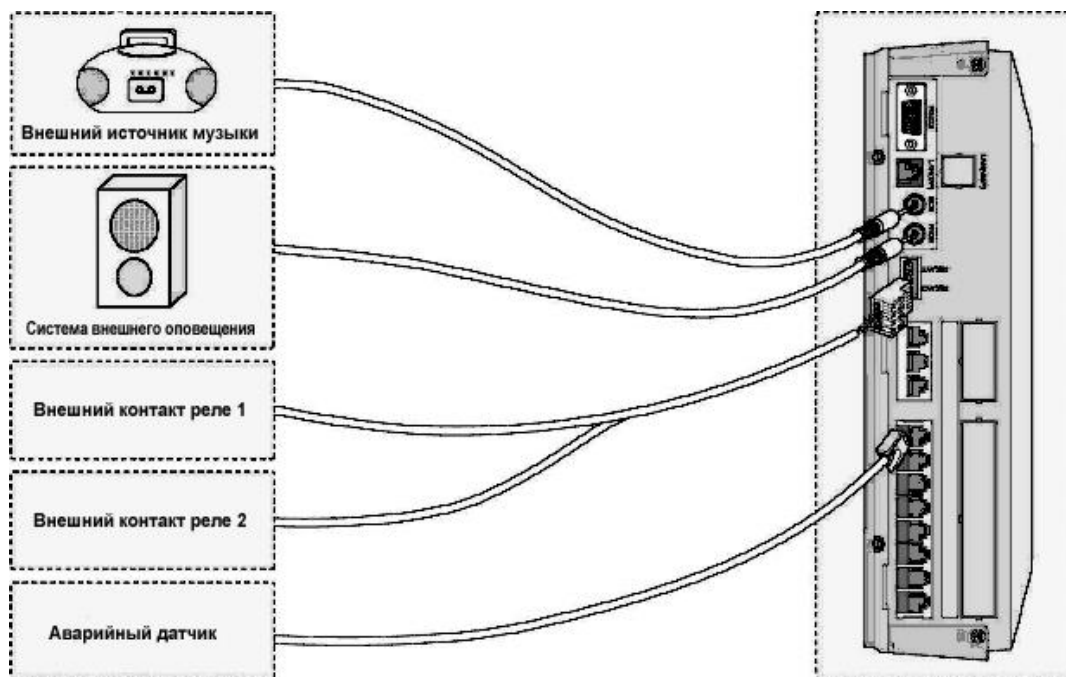
Рис. 5.1.3 Подключение дополнительных устройств
