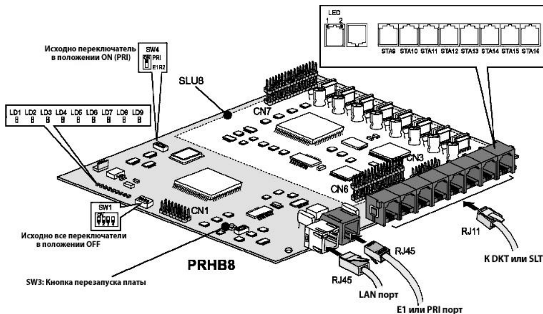
Рис. 4.4.6 PRHB8
