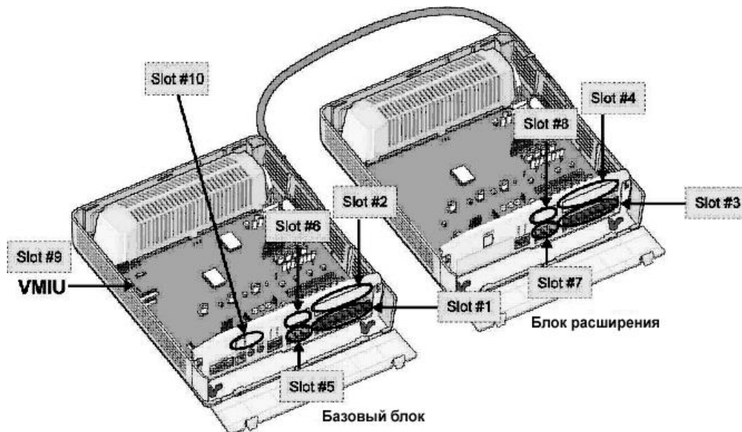
Рис. 6.2.3.2 Расположение платомест
