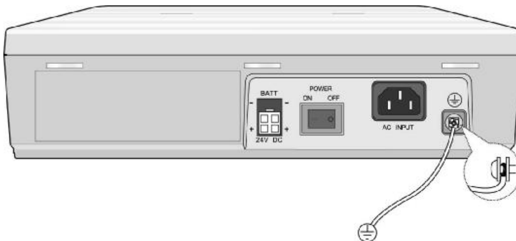
Рис. 3.2.5 Заземление корпуса
