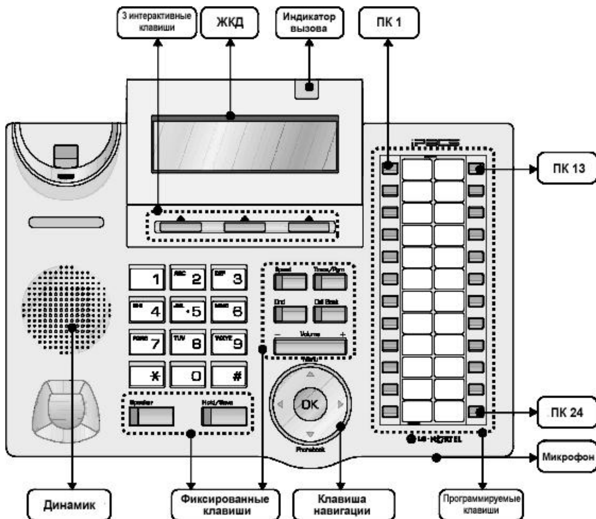
Рис. 6.2.1.2 Описание клавиш IP телефона LIP-7024D
