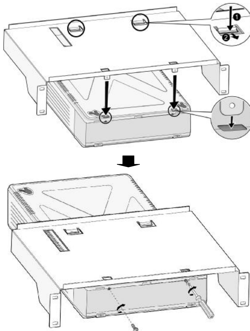
Рис. 3.3.3.2а Установка стоечного крепления
