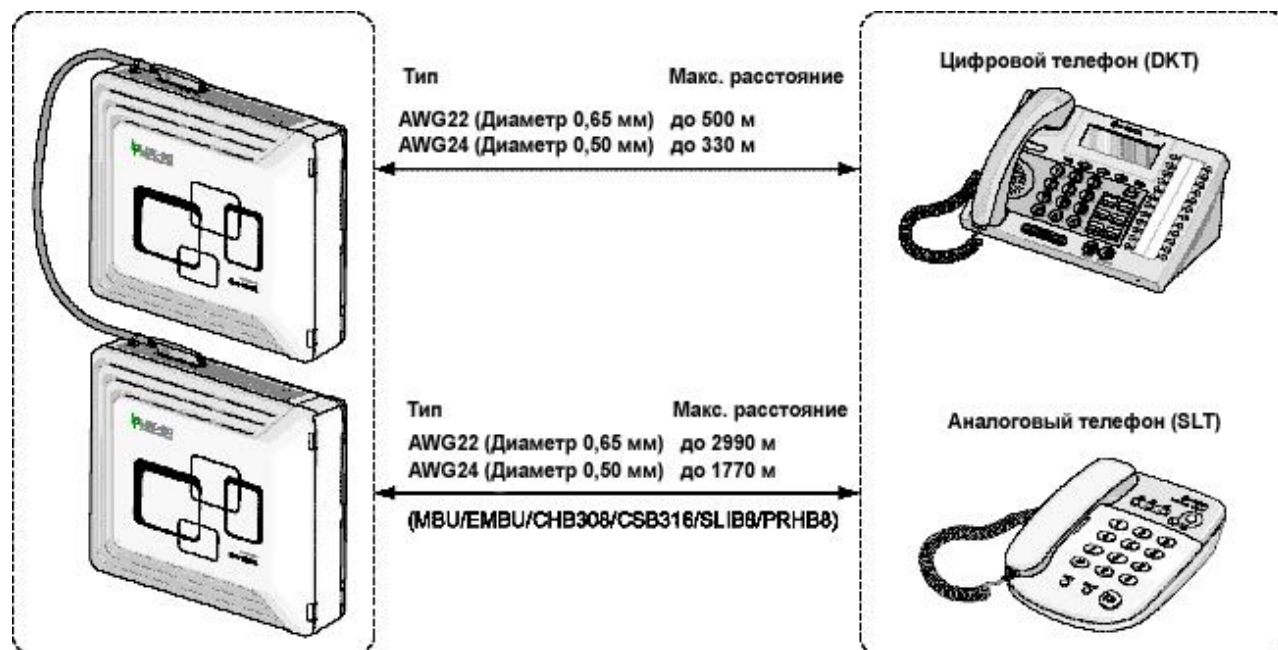
Рис. 5.1.1 Максимальная удаленность терминалов
