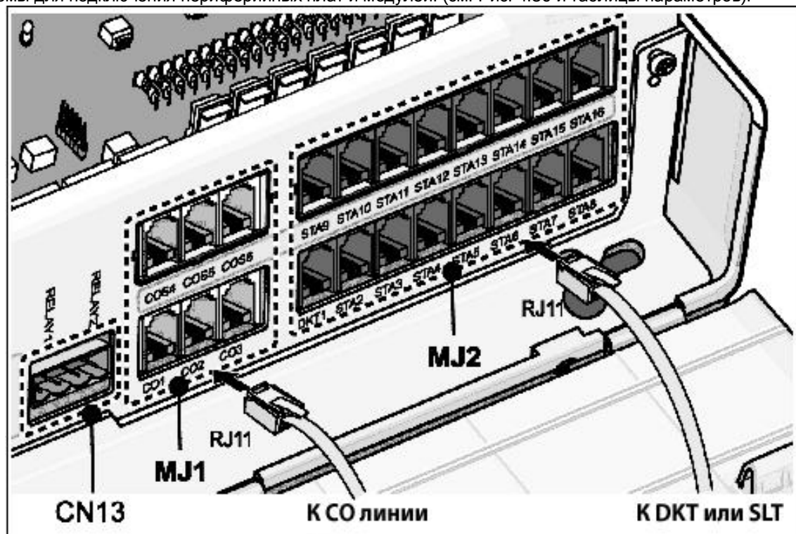
Рис. 4.36 Подключение
