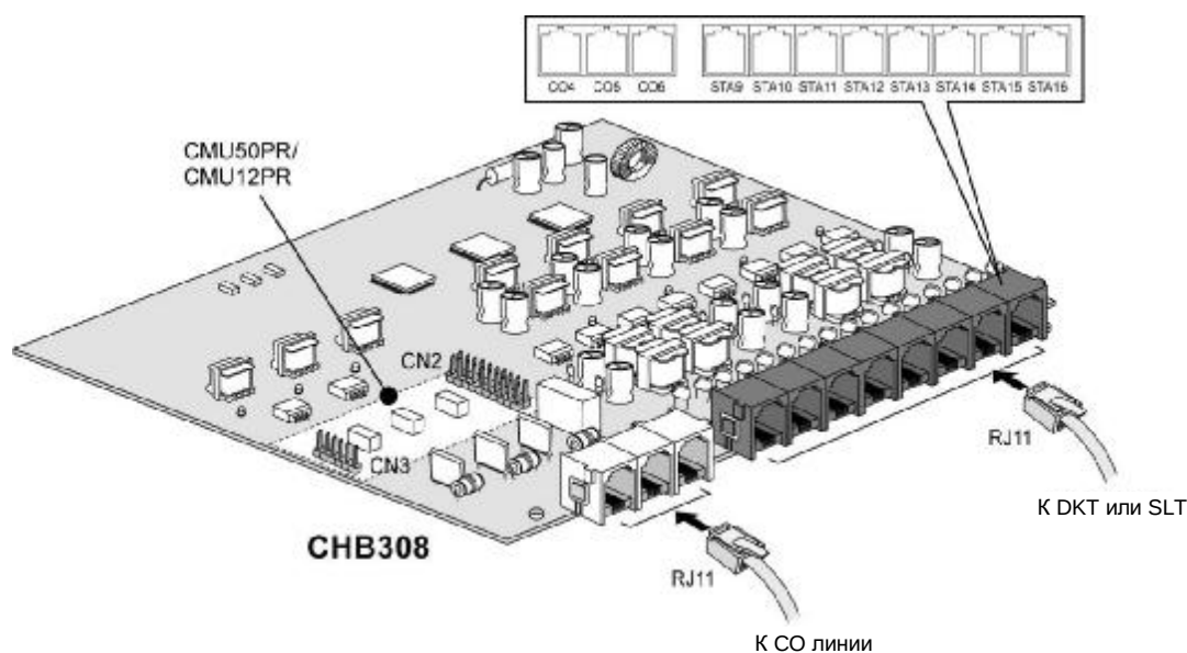
Рис. 4.4.1 CHB308
