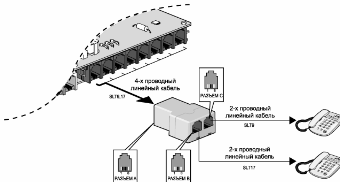
Рис. 4.4.2.2 Терминальный переходник
