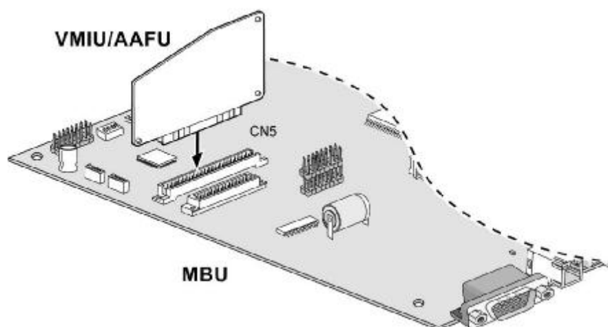
Рис. 4.5.1 VMIU/AAFU
