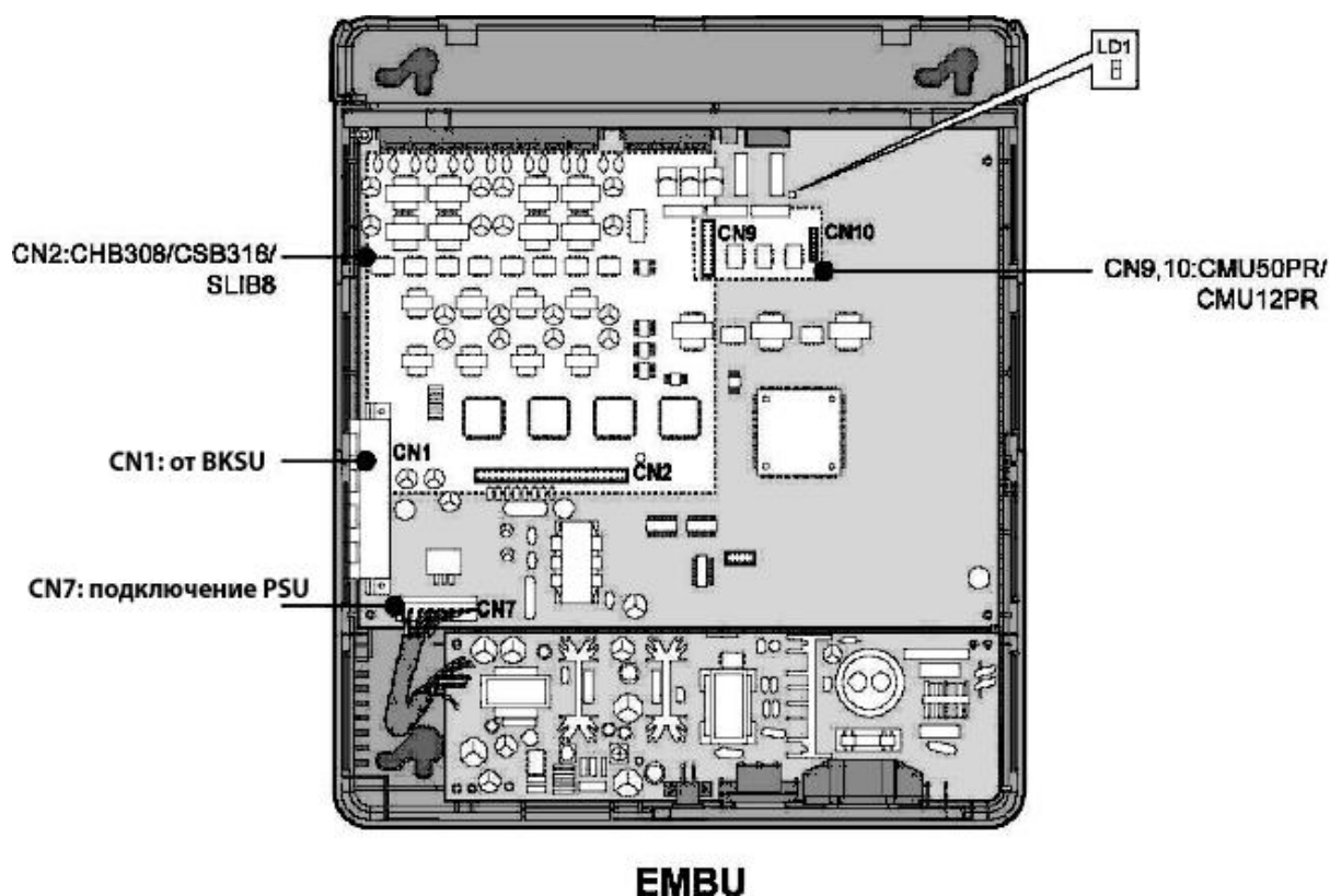
Рис. 4.3а Материнская плата блока расширения (EMBU)
