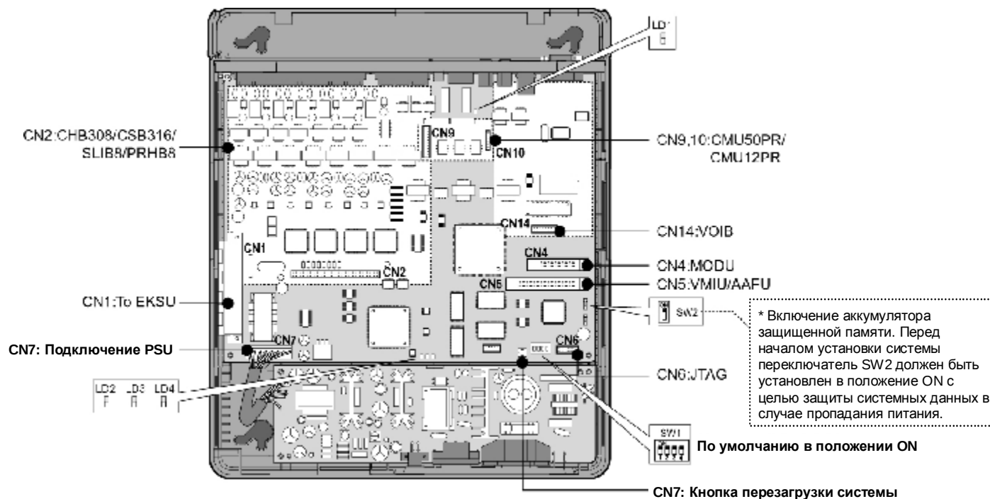
Рис. 4.2а Материнская плата базового блока (MBU)
