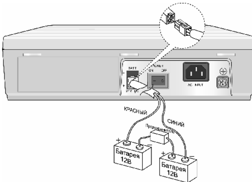
Рис. 3.2.6 Подключение внешних резервных батарей
