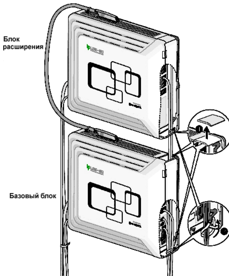
Рис. 5.2.1 Прокладка кабелей при настенном монтаже
