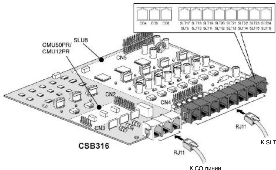
Рис. 4.4.2.1 CSB316
