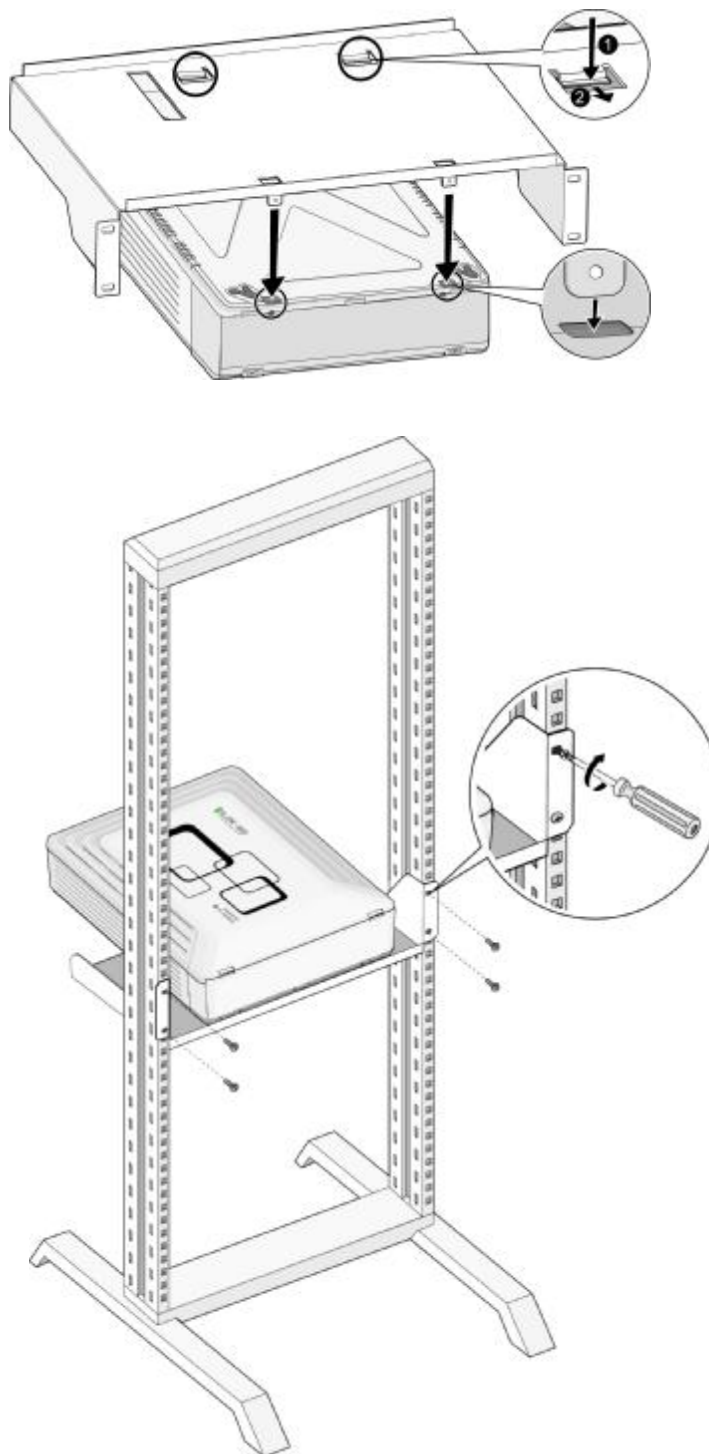
Рис. 3.2.7.2 Монтаж системного блока в стойке
