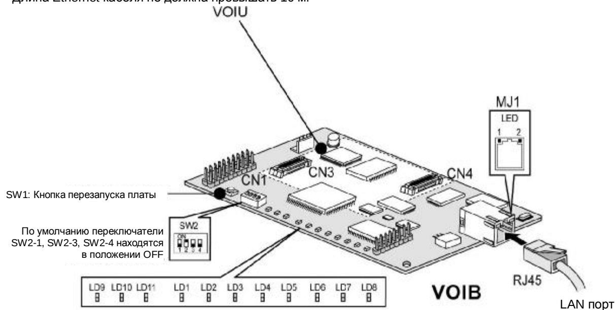
Рис. 4.4.4 VOIB
