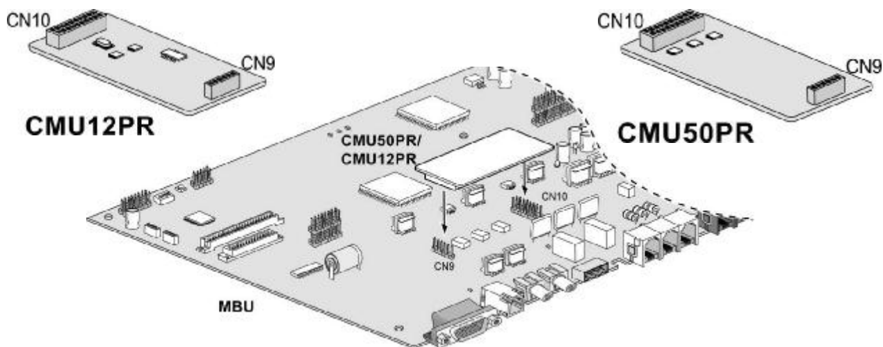
Рис. 4.5.6 CMU12PR и CMU50PR
