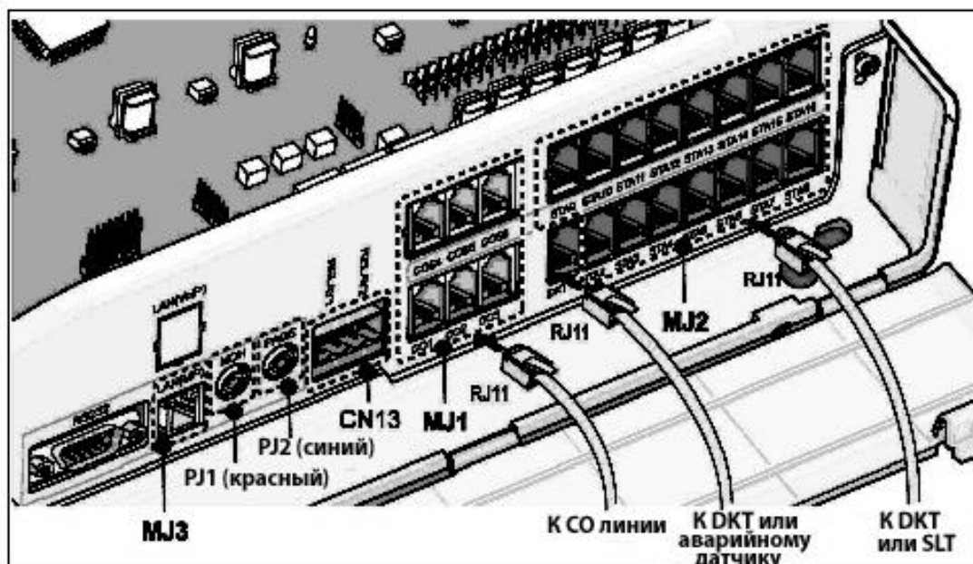
Рис. 4.26 Подключение по портам
